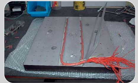
Hier werden neue Heizpatronen montiert und elektrisch verdrahtet.
