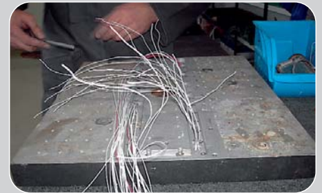
Hier zeigen wir am Beispiel einer „Sandwich-Vorheizung“ wie eine Überholung bei TEFTEC aussieht. Das stark reparaturbedürftige Werkzeug mit verschlissener Beschichtung.
